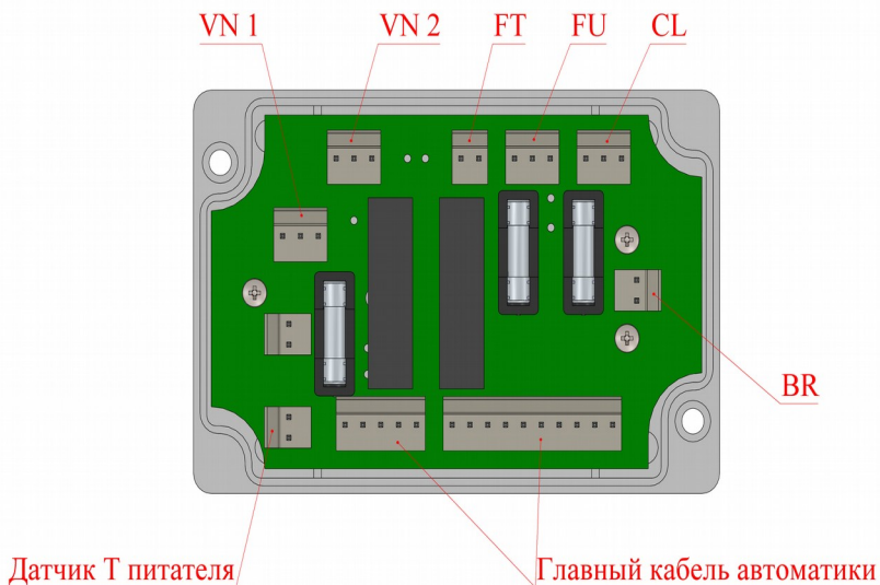
Рис.4 Схема подключений в блоке коммутации горелки KVIТ Optima R
