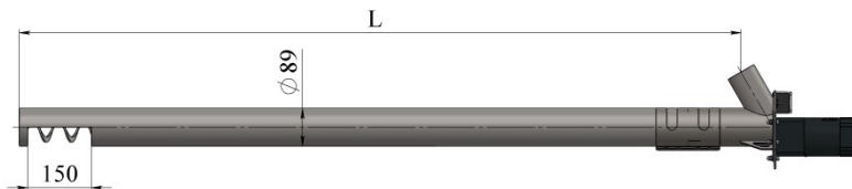
Рис.2 Геометрия комплектного шнека KVIТ Optima
